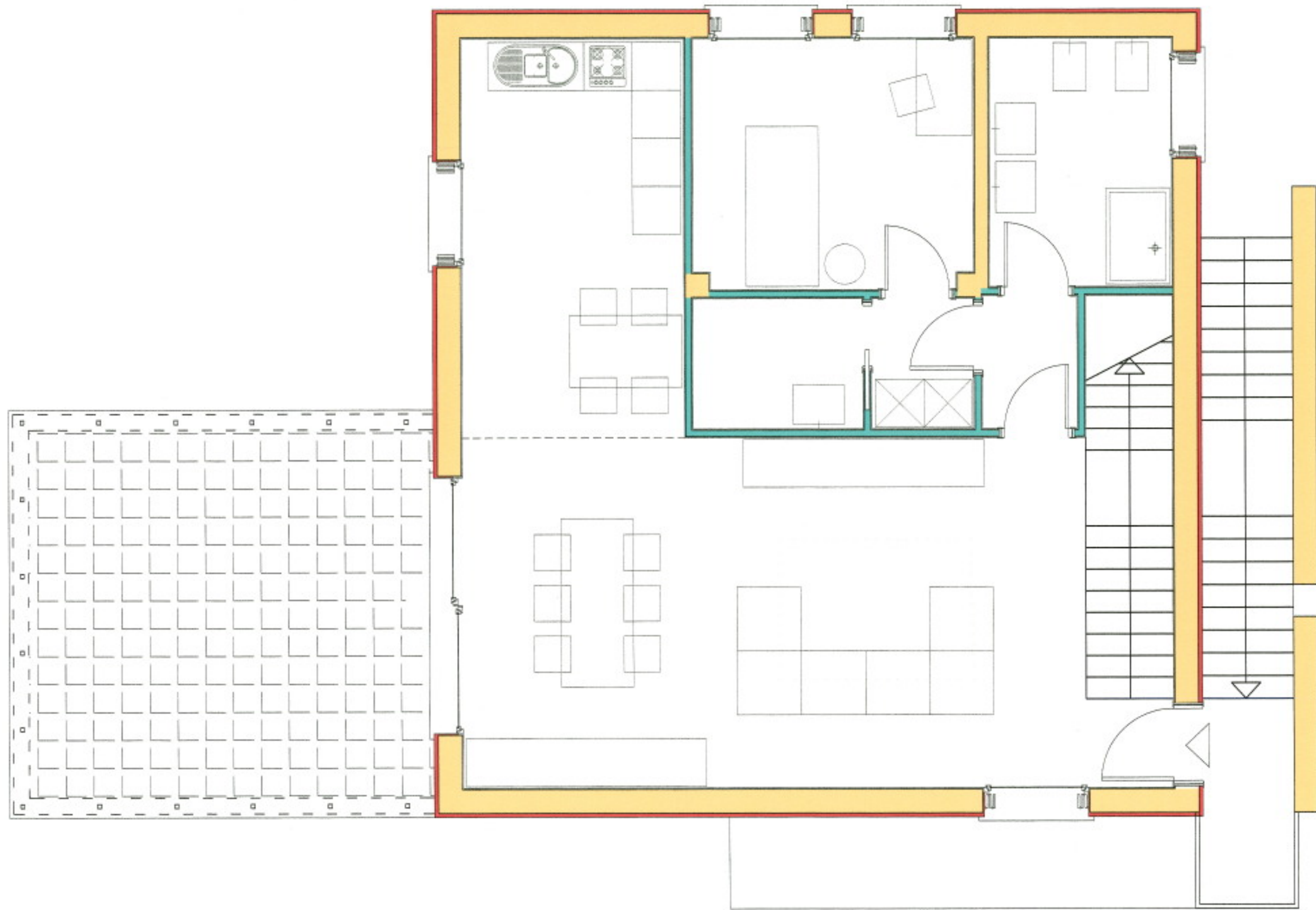
BLOCCO B PLANIMETRIA PRIMO PIANO
